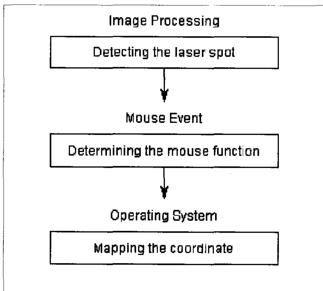
그림 7. 소프트웨어 구성
